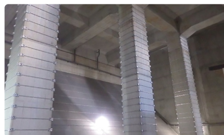
高架橋の柱に対する耐震補強②
