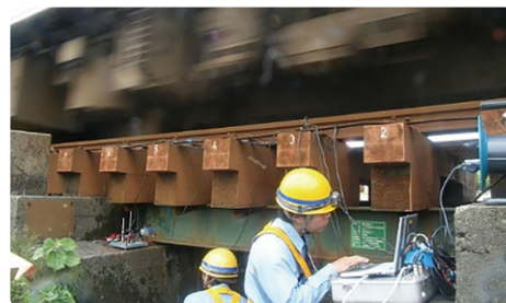
検査機器を用いた橋りょうの詳細検査
